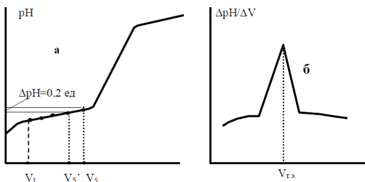
Рис. 4-4. Кривые титрования
