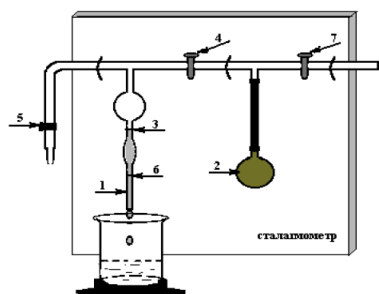
Рис. 5-1. Устройство сталагмометра
